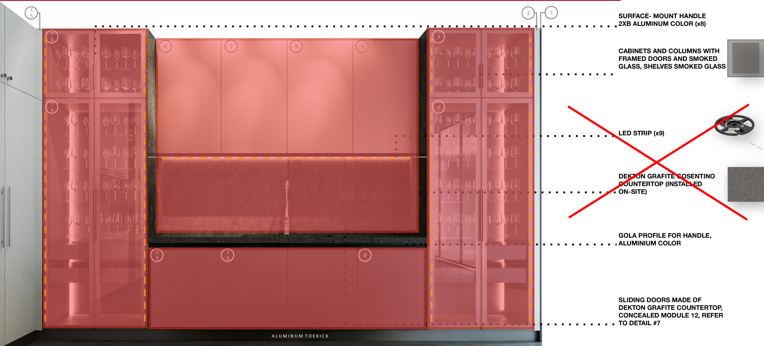
ELEVATION A
