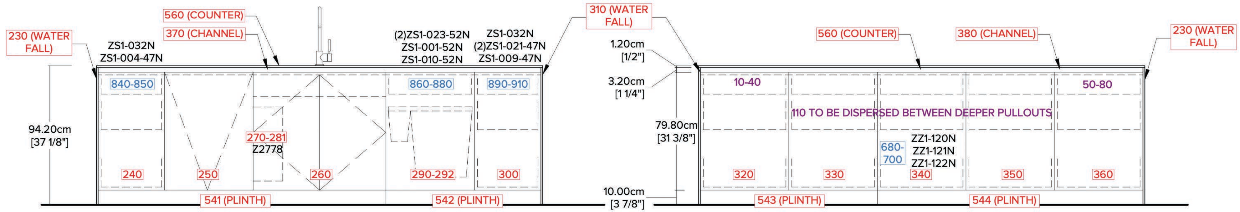
B ELEVATION
