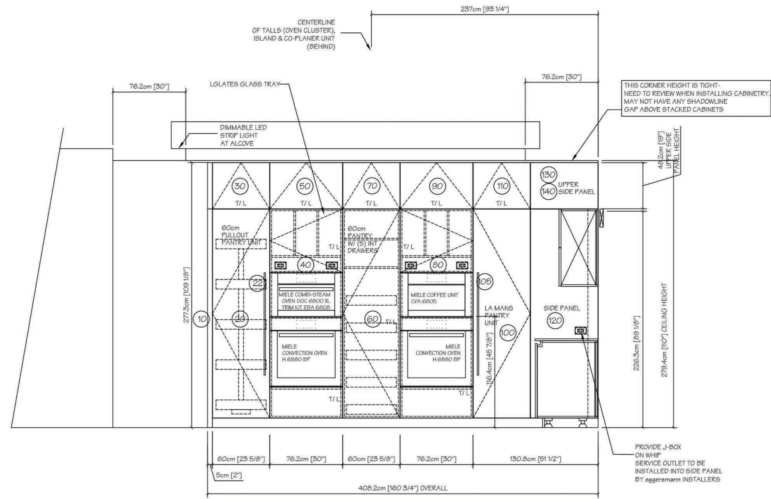
ELEVATION A
