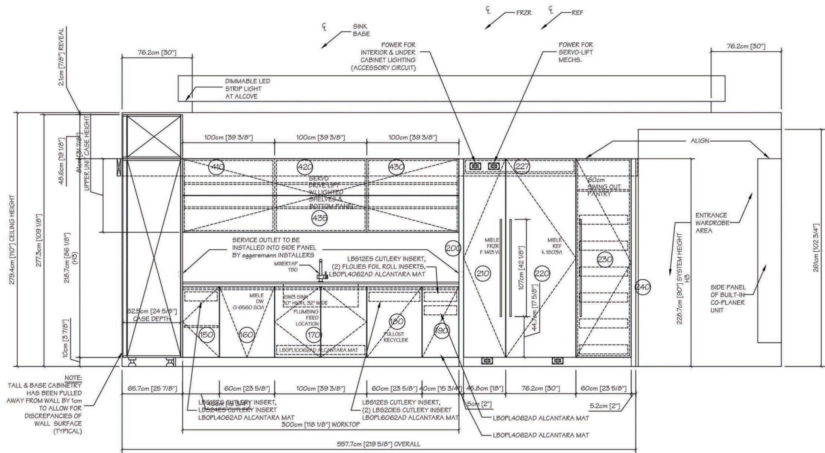
ELEVATION B
