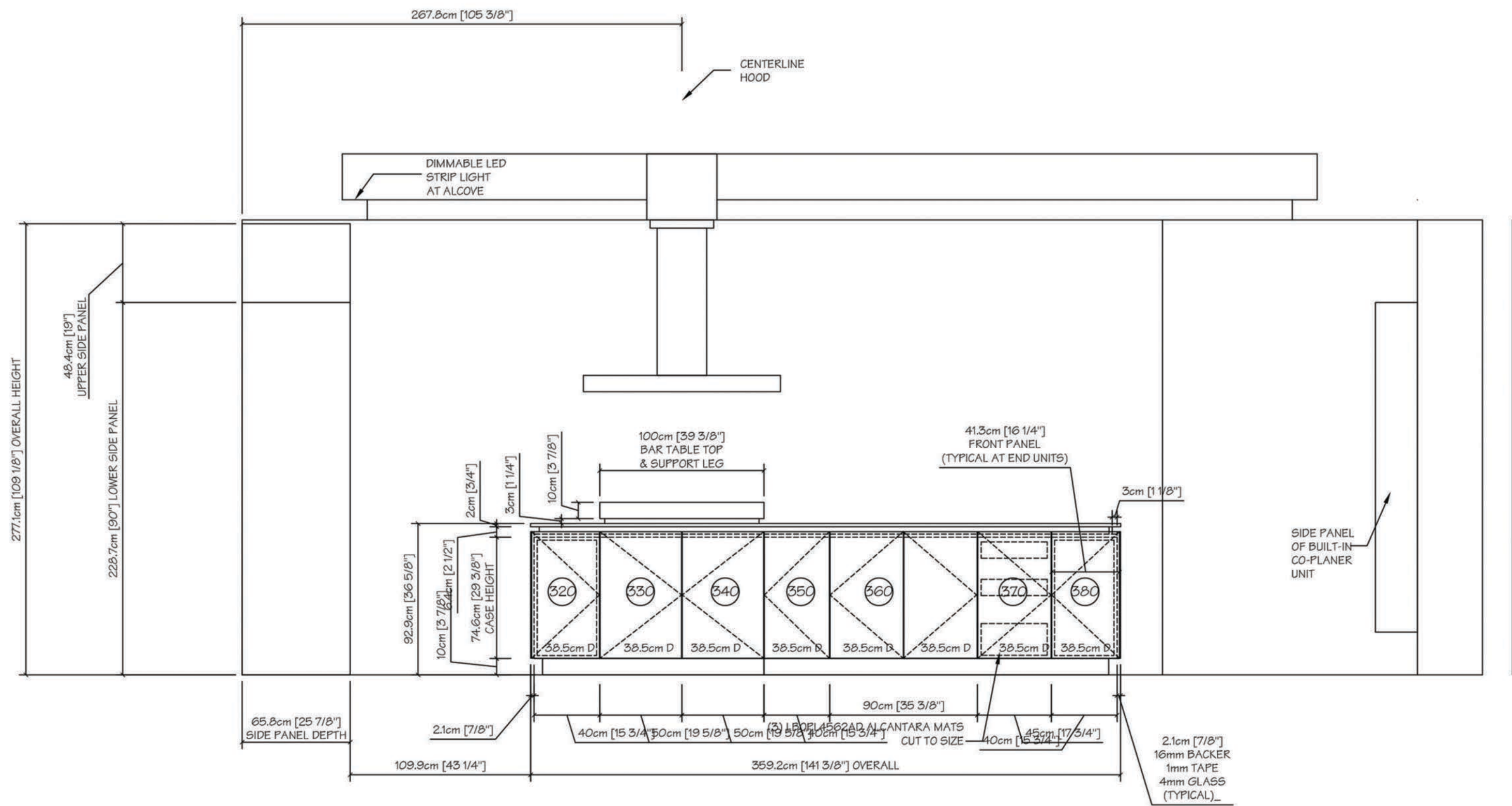
ELEVATION E
