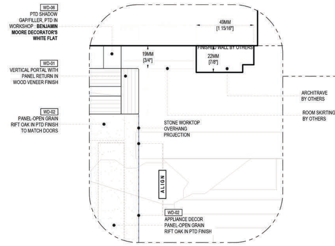
2 DETAIL-02 SCALE: 6" = 1'-0"
