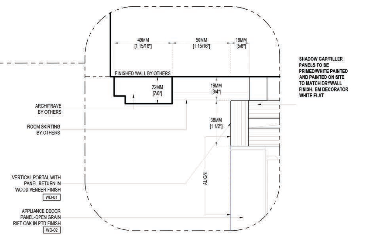
1 DETAIL-01 SCALE: 6" = 1'-0"
