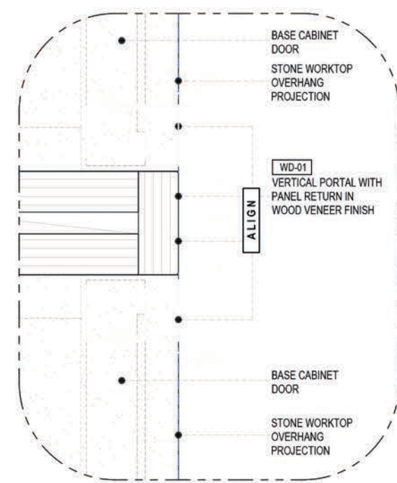
3 DETAIL-03 SCALE: 6" = 1'-0"
