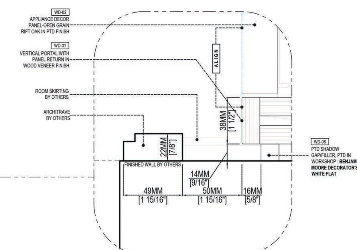
3 DETAIL-03 SCALE: 6" = 1'-0"
