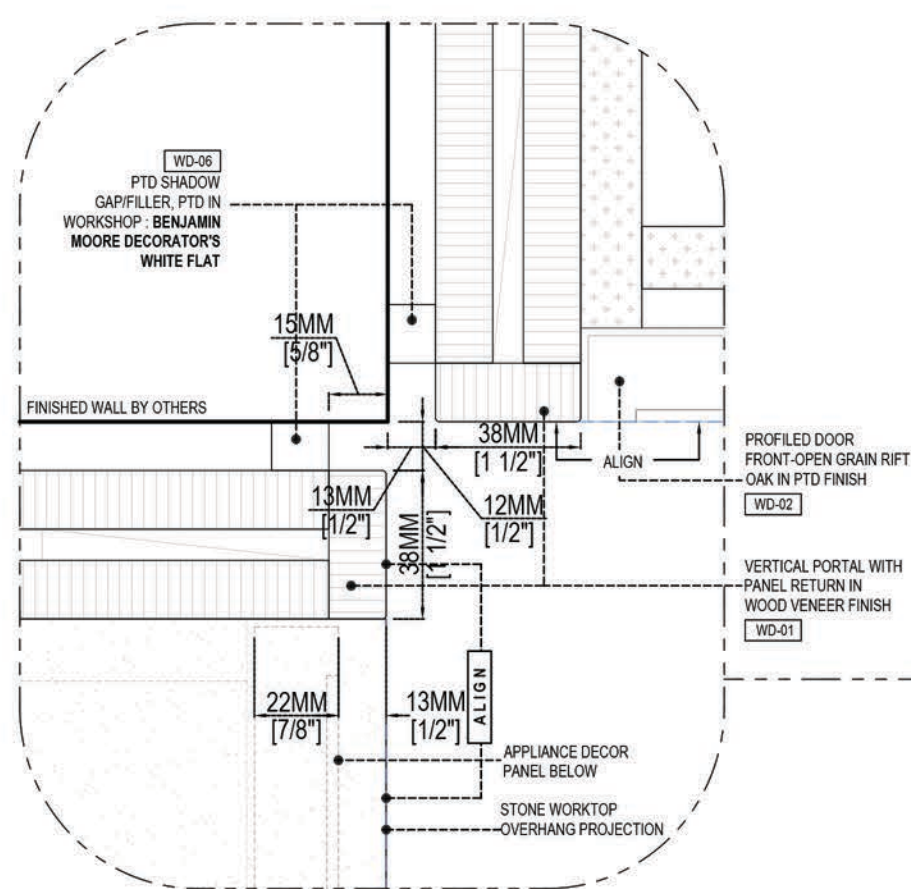
1 DETAIL-01 SCALE: 6" = 1'-0"
