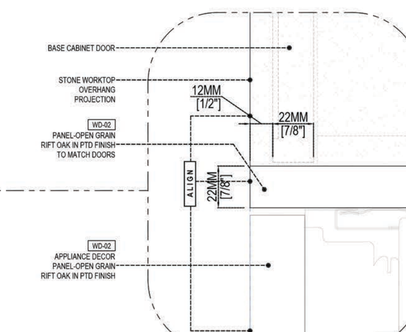
2 DETAIL-02 SCALE: 6" = 1'-0"
