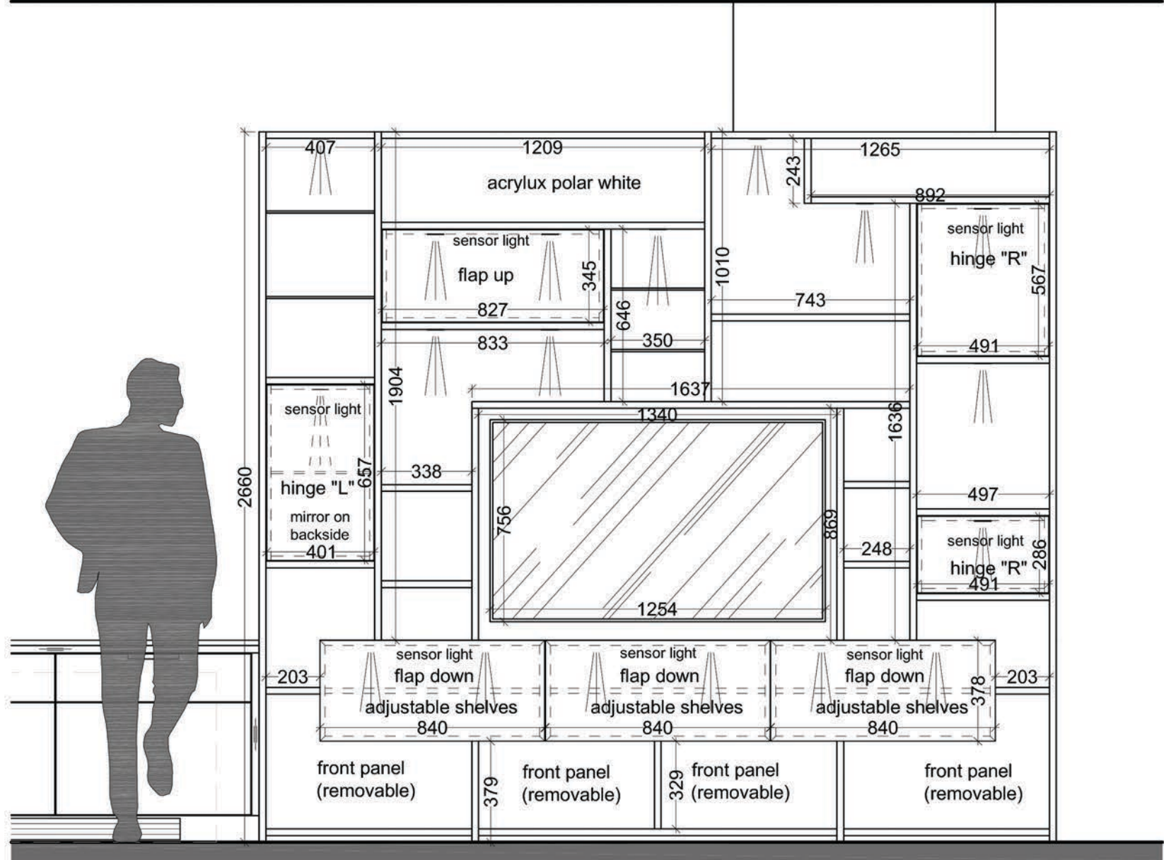
elevation A
