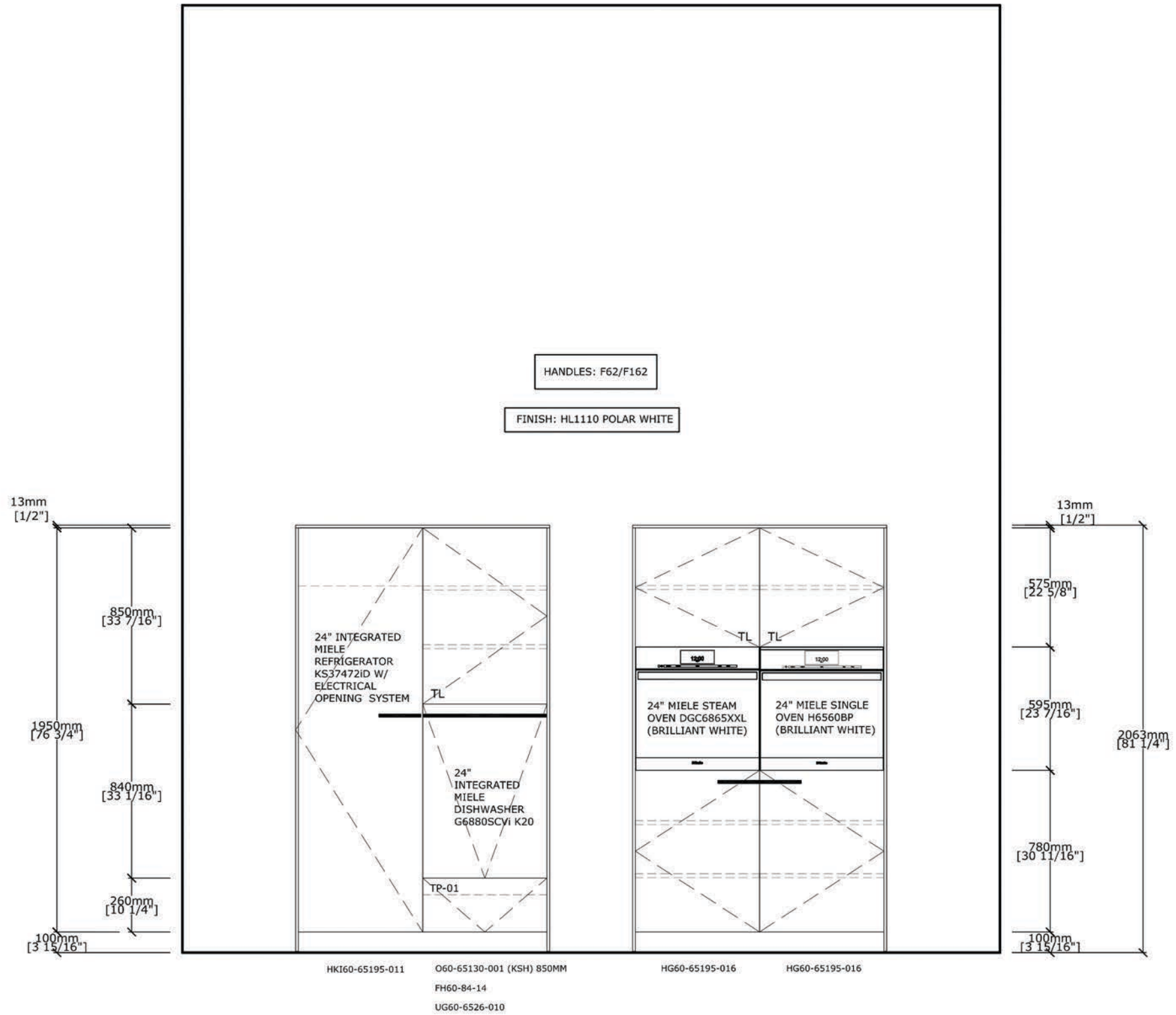
A VENOVO DISPLAY ELEVATION
