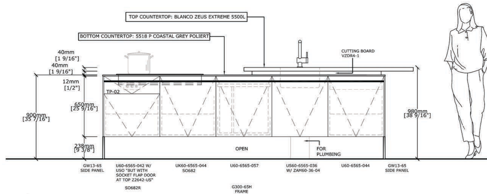
B VENOVO DISPLAY ELEVATION
