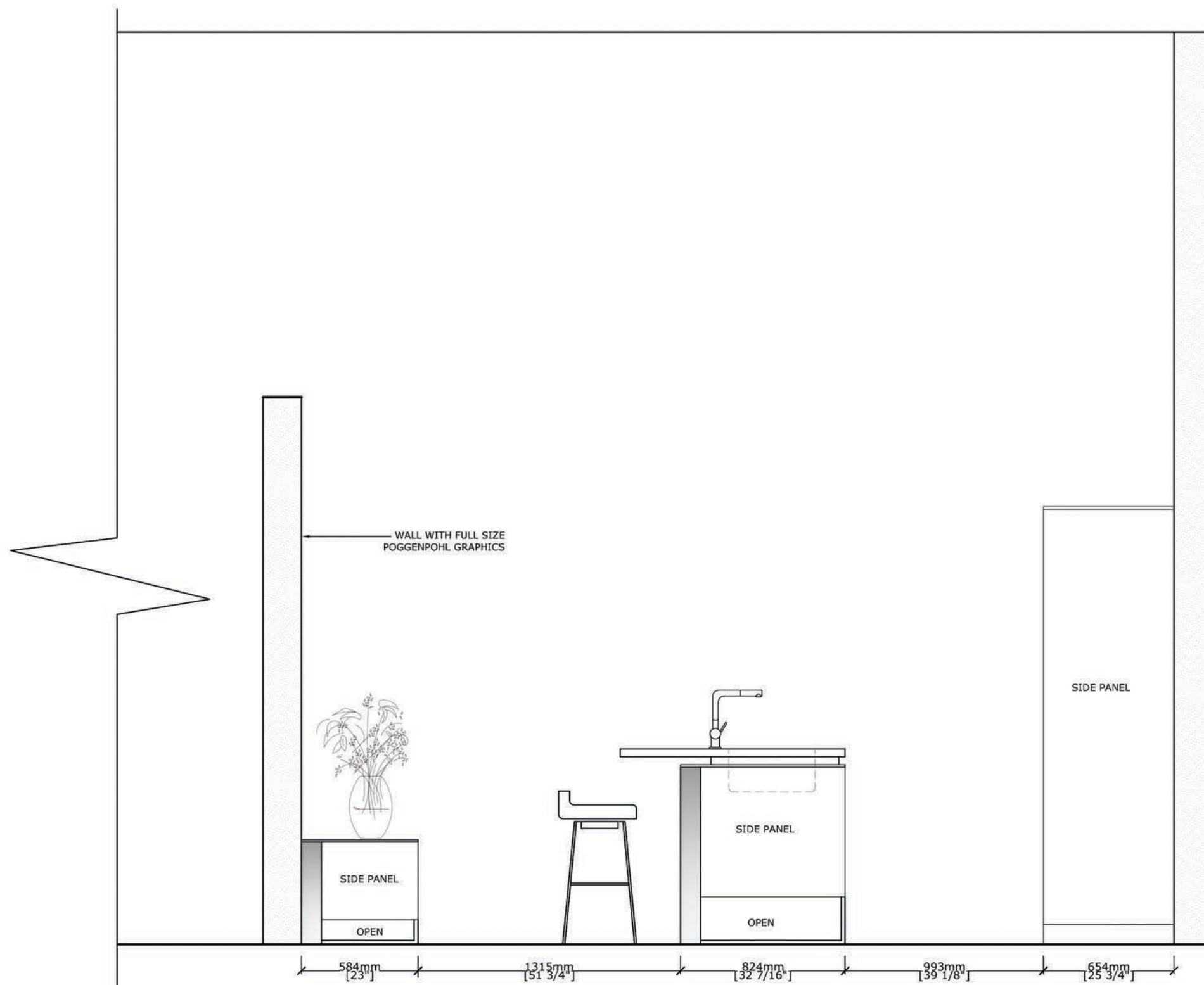
C VENOVO DISPLAY ELEVATION
